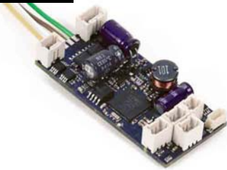
Der LS Standardtyp, beispielbar mit diversen Soundprojekten Standard LS type, programmable with various sound projects
